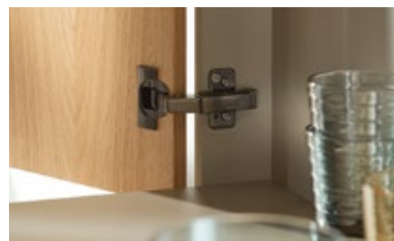
CLIP top BLUMOTION под фальшпанель, вкладная петля
